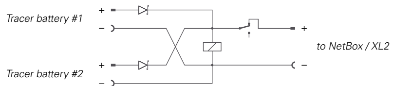
Blockdiagramm Tracer-Batterie Adapterkabel
