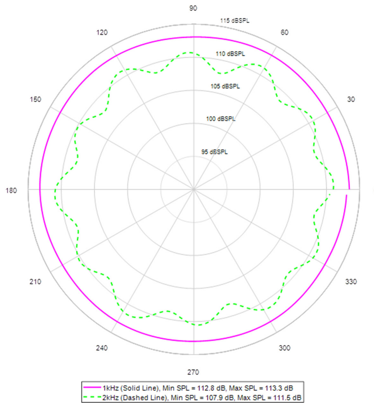
Polardiagramm des DS3 bei 1 kHz und 2 kHz in der horizontalen Ebene, gemessen mit Terzanalyse in 1.5 m Distanz (Anregungssignal: GlideSweep)
