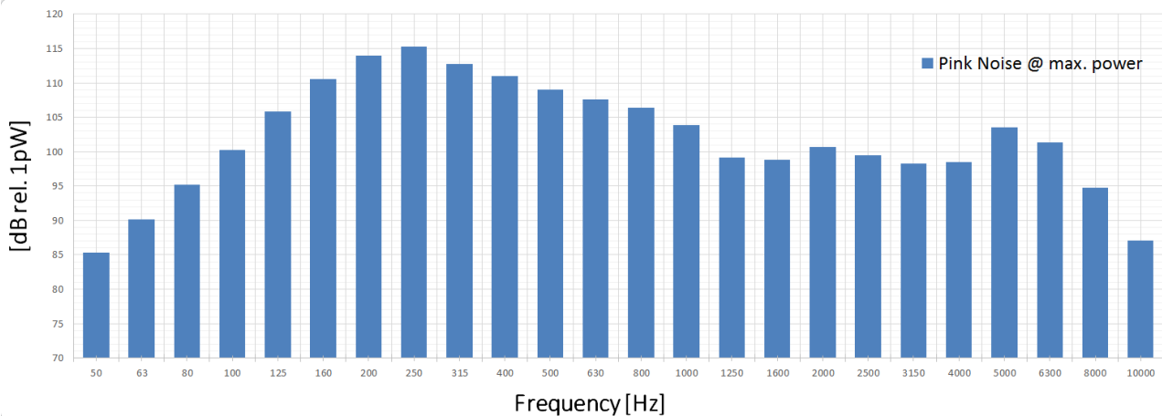
Frequenzgang des DS3 bei PA3 Einstellung 'Pink (max. Schalleistung)
