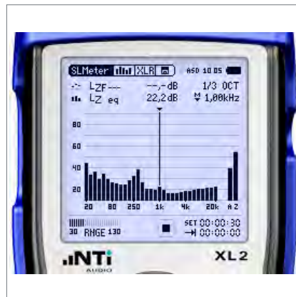
Spektrum des Hintergrundgeräuschpegels im Empfangsraum
