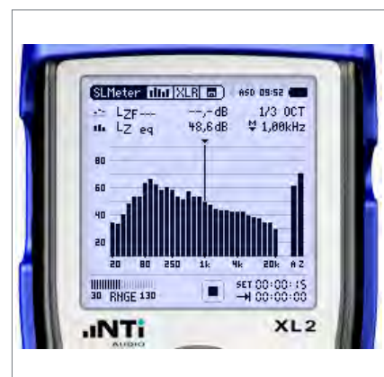
Geräuschspektrum im Empfangsraum
